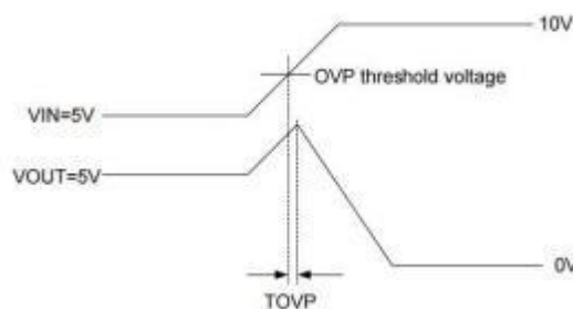
过压保护响应时间测试图
