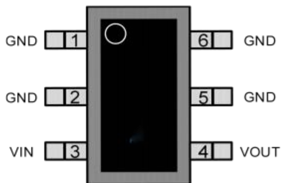
SOT23-6L
